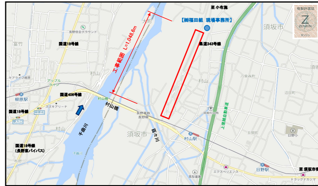
施工場所位置図
